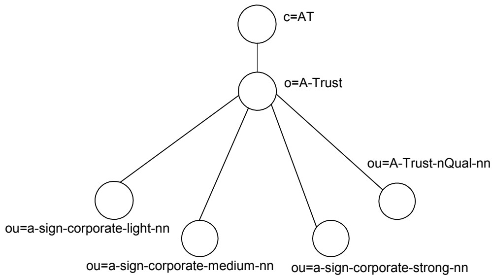
Abbildung 2 a.trust Verzeichnisbaum
