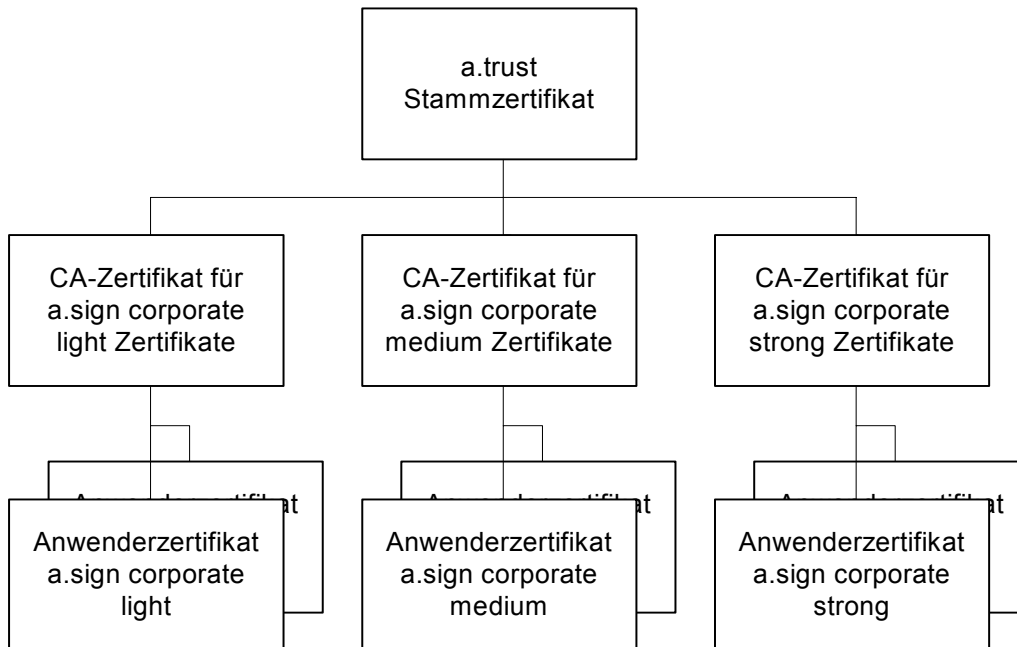
Abbildung 1 Zertifizierungshierarchie
